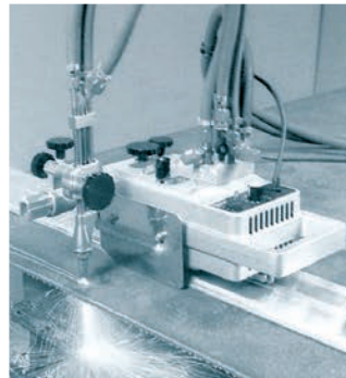
ProFIT für automatische Geradeschnitte durch Laufbahnführung
