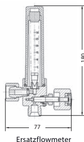
Ersatzflowmeter
