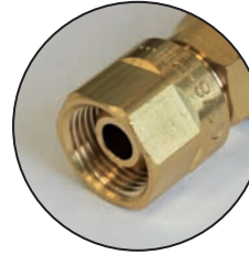
Standardschlauchan- schluss nach EN 560. Markierung für einfache Erkennung der Anschlussmaße.
