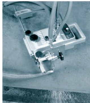
ProFIT mit einseitig angeordneten Brennern für Schweißkantenschnitte
