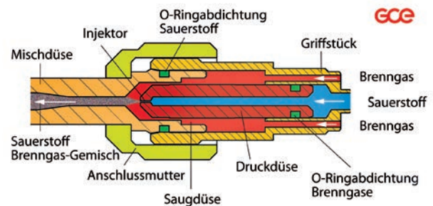
PROFI S 89 INJEKTOR
