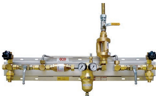
Acetylen-Versorgung
